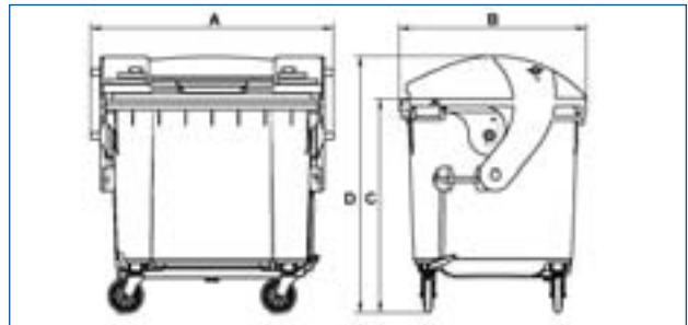
Ausführung mit Schiebedeckel, Maße siehe Tabelle
