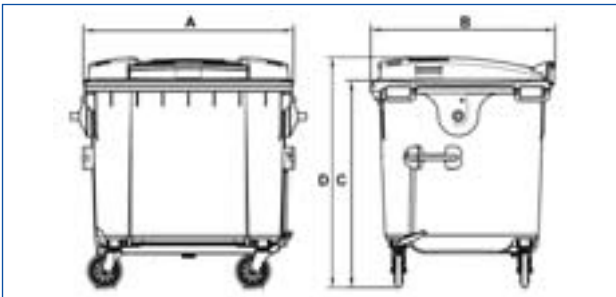
Ausführung mit Flachdeckel, Maße siehe Tabelle
